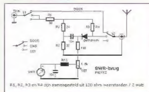
Figuur 6. Het schema van de tien jaar oude kleine meter, met draaischakelaar.
